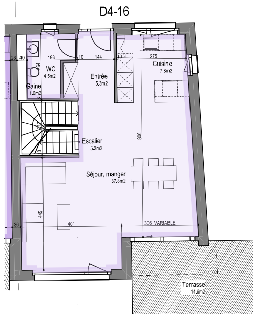
REZ-DE-CHAUSSEE
