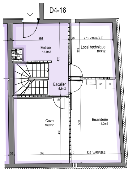
SOUS-SOL
