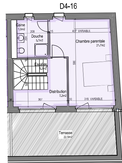
ETAGE 2
