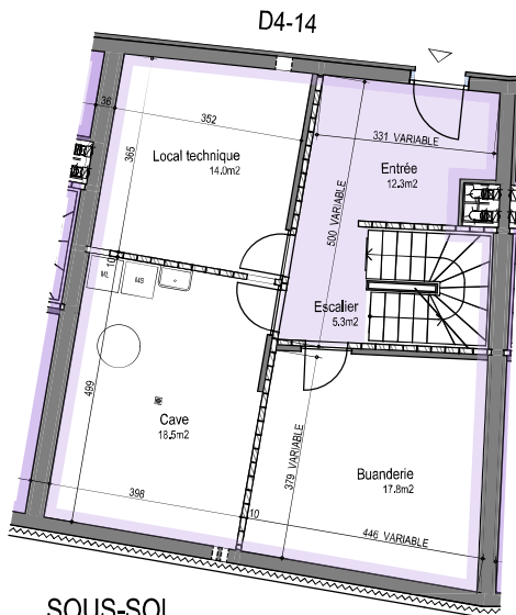
SOUS-SOL
