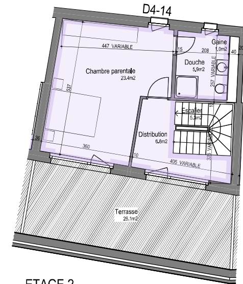
ETAGE 2
