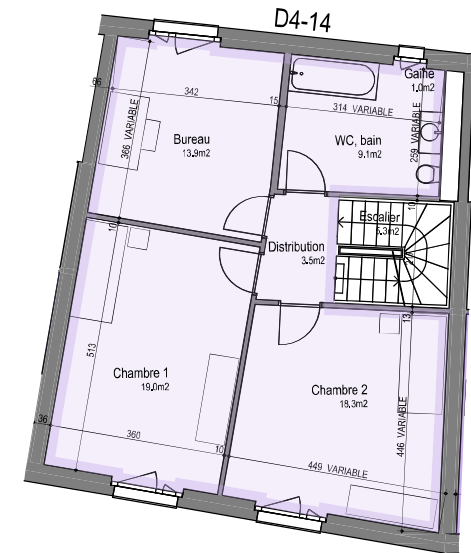
ETAGE 1
