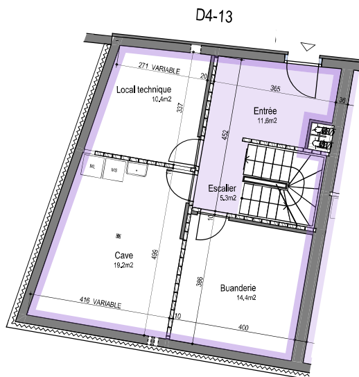
SOUS-SOL
