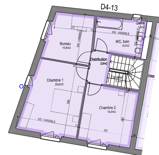
ETAGE 1
