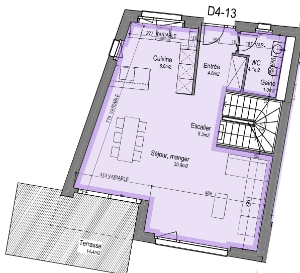
REZ-DE-CHAUSSEE
